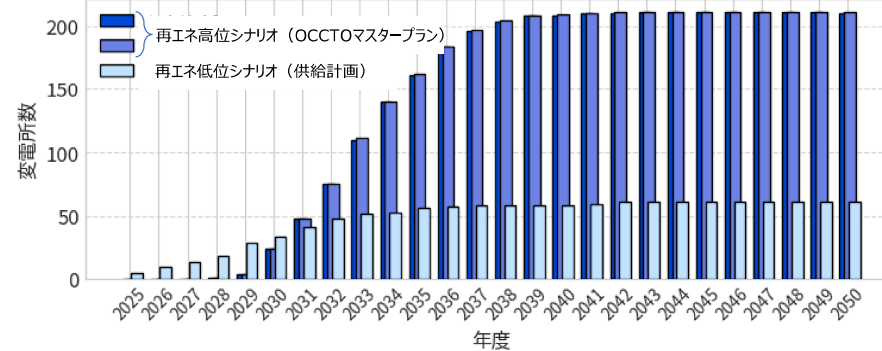
逆潮流により過負荷が発生する変電所数（東京電力PGの例）
