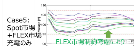
各DER運用シナリオに対する電圧挙動
