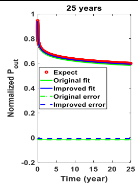
図 2 開発した劣化挙動予測モデルによる 25 年間の出力予想結果例。
