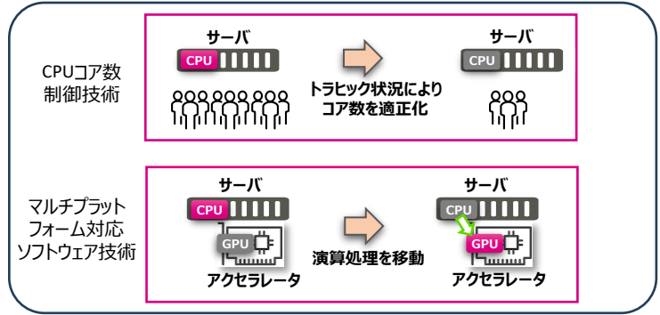
CU/DU向け省電力技術
