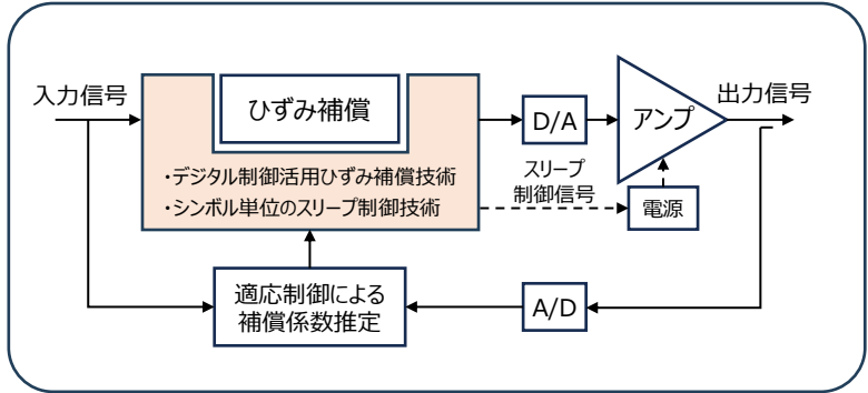
RU向け省電力技術
