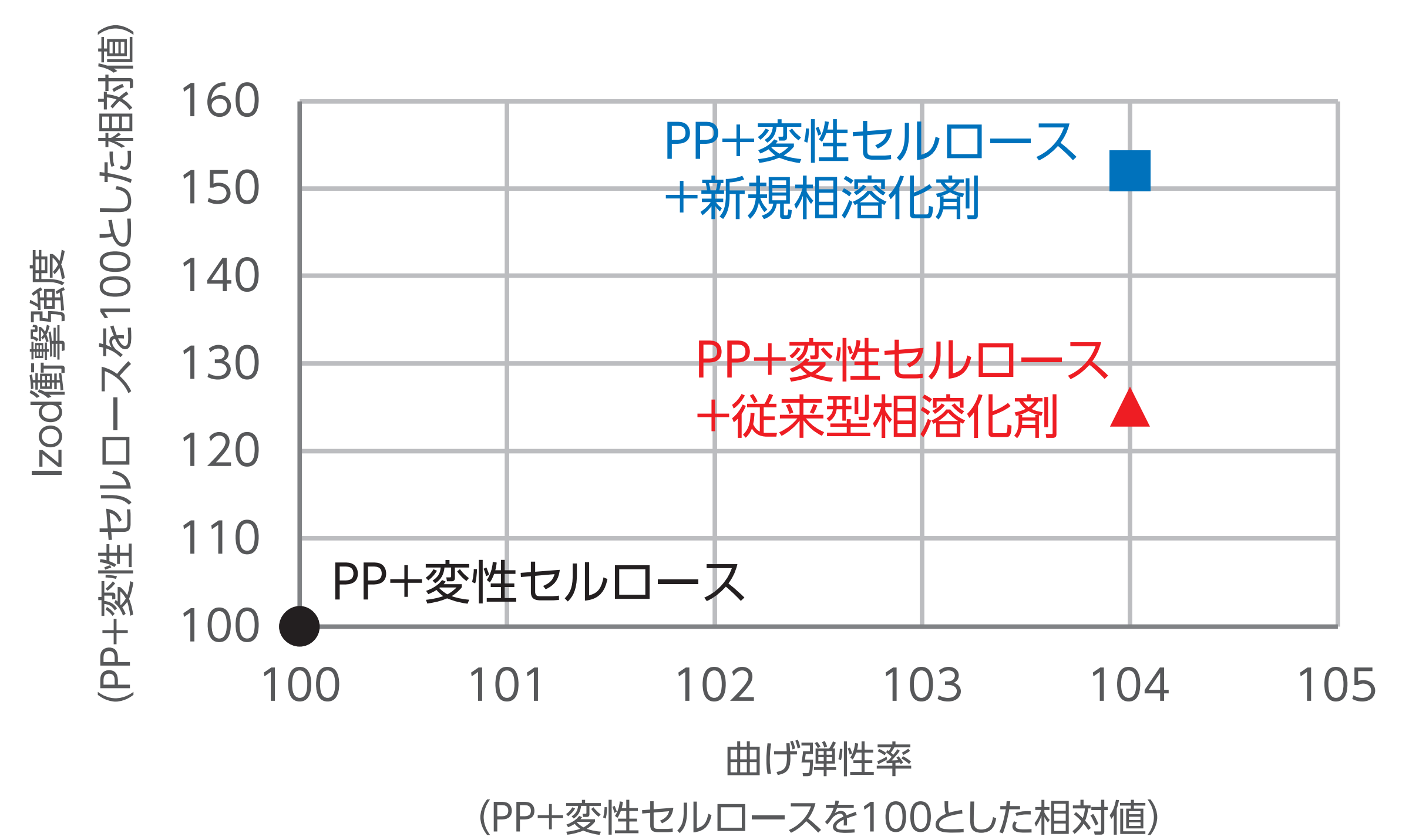
図3 CNF複合材料の曲げ弾性率と衝撃強度の関係
