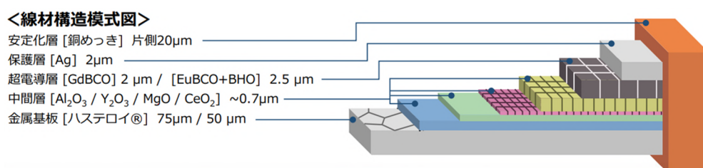
図 3-5-18 REBCO 線材の構造模式図
