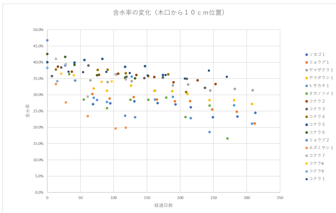
図3 含水率の推移
